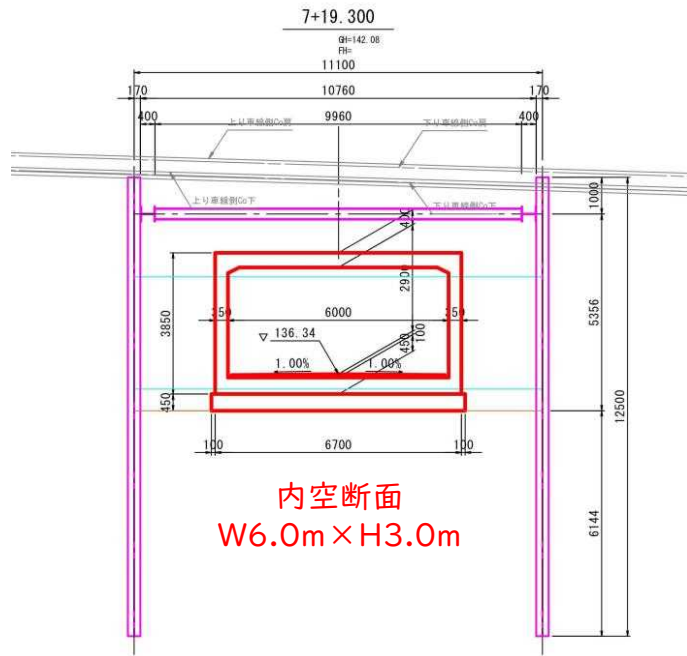
計画横断面図
