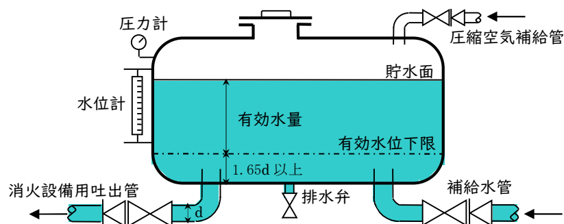
第2-14図 圧力水槽の場合
