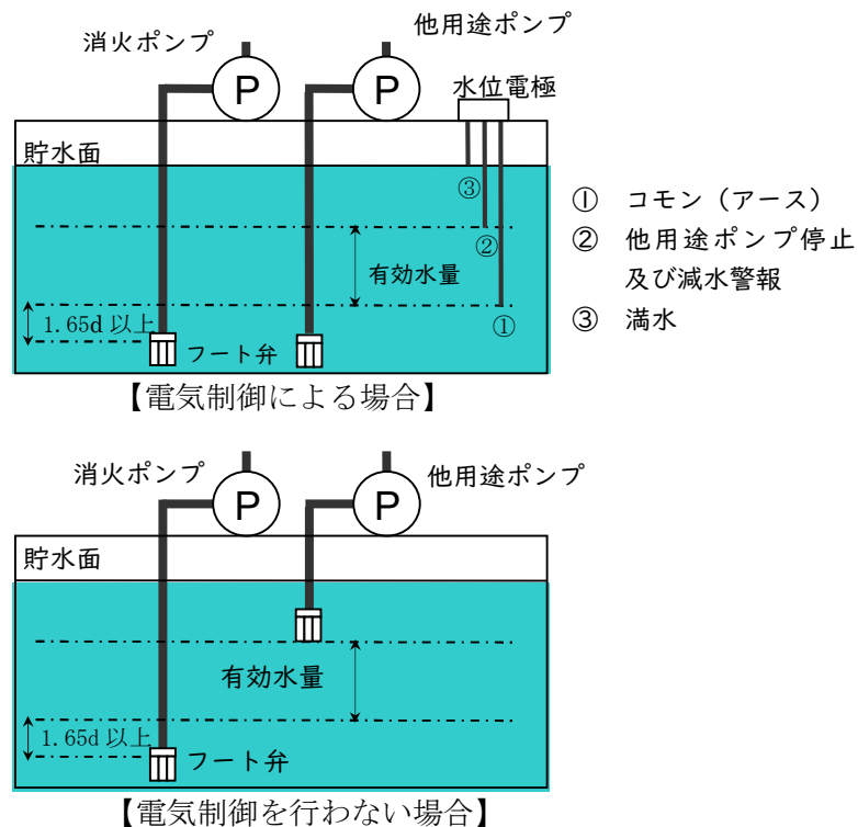
第 2-13 図 地下又は床下水槽の場合
