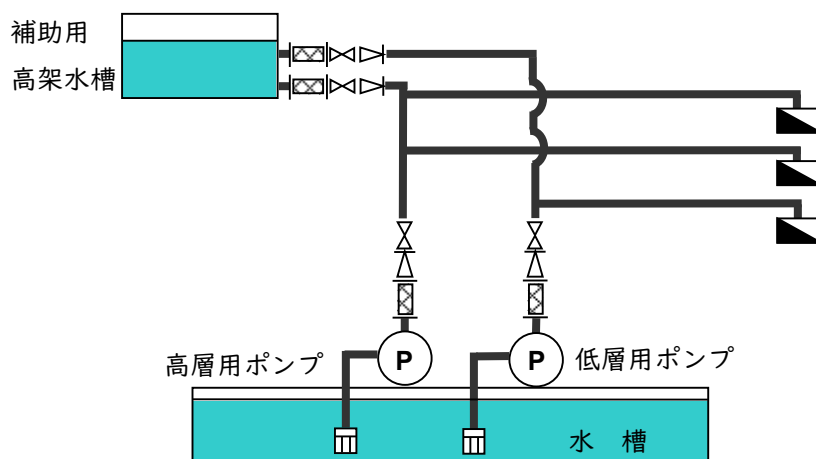
第2-6 図 ポンプ揚程を考慮し配管を別系統にする方法の例
