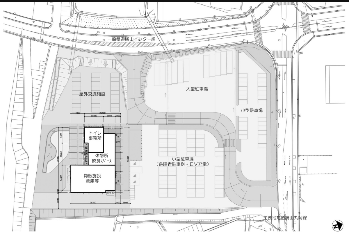
道の駅計画平面図
