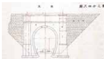
隧道図正面
