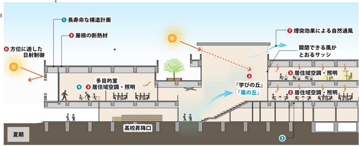
『学びの丘』の自然通風など、パッシブデザインによる環境負荷
