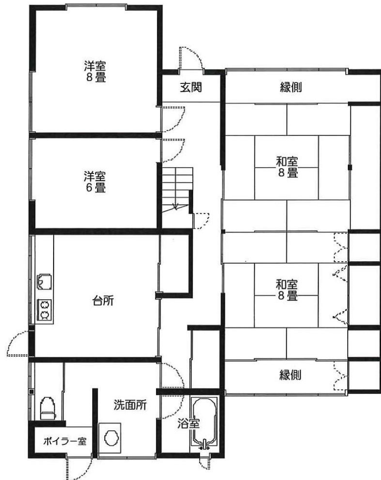
1 階平面図
