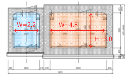
断面②
