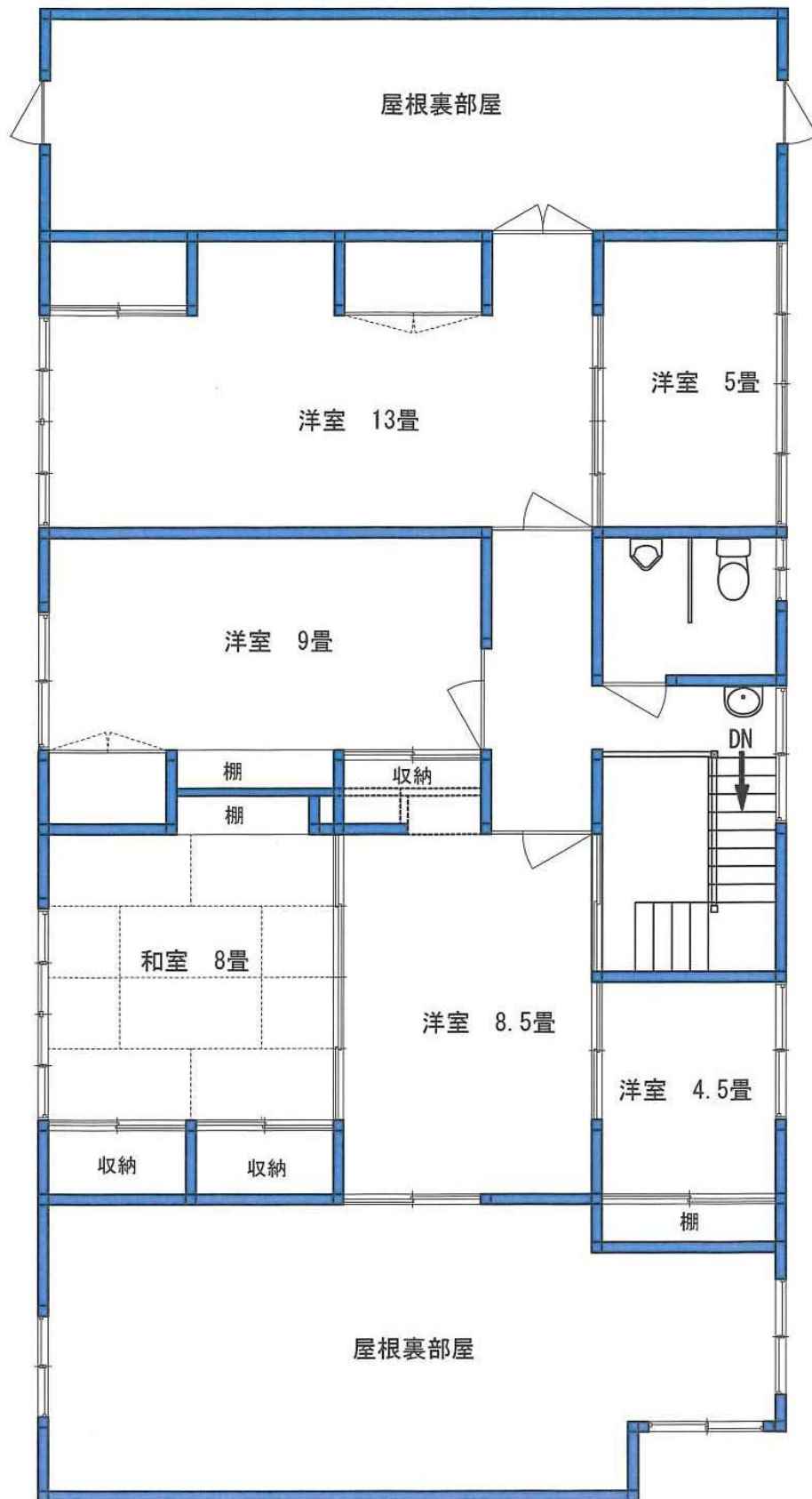
2 階 平 面 図
