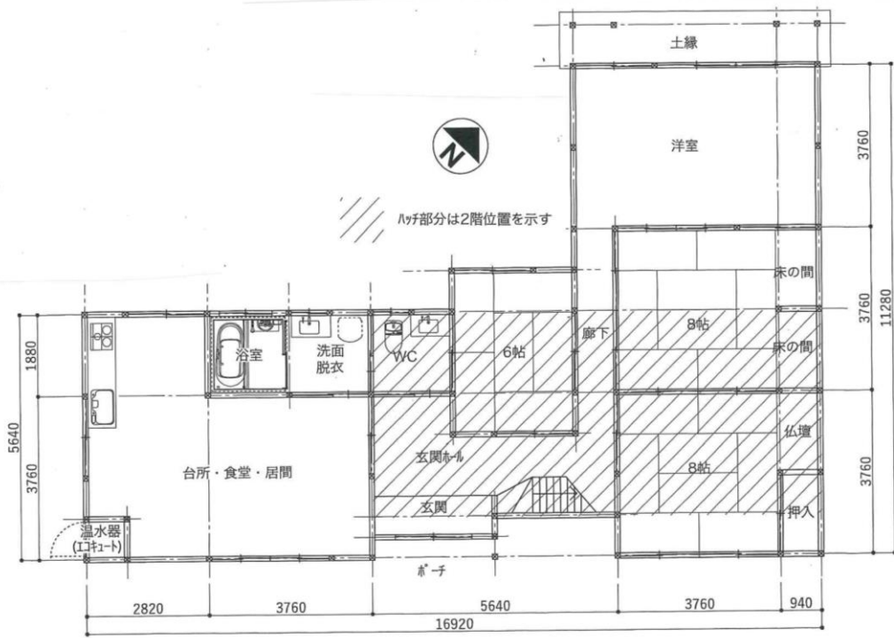
1階平面図
