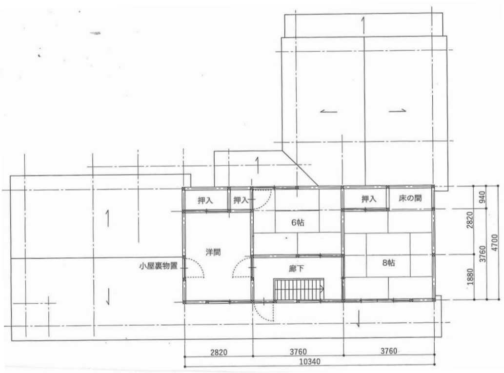
2階平面図
