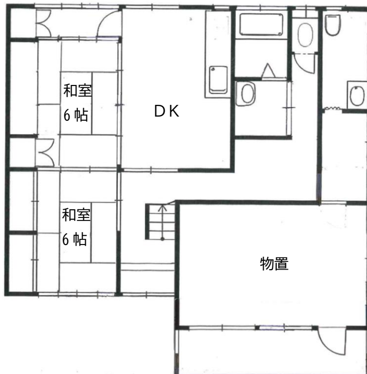
1階平面図
