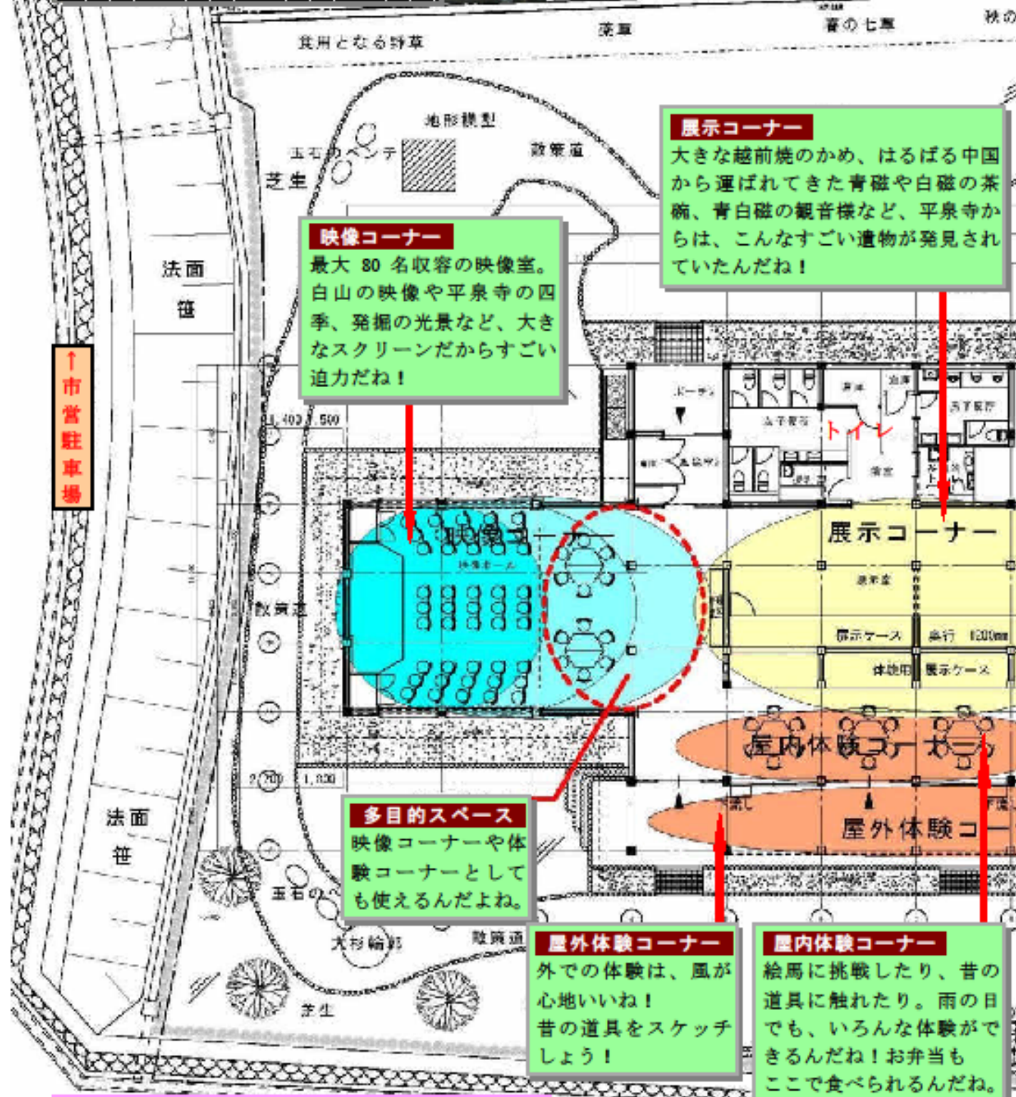
史跡ガイダンス施設計画平面図
